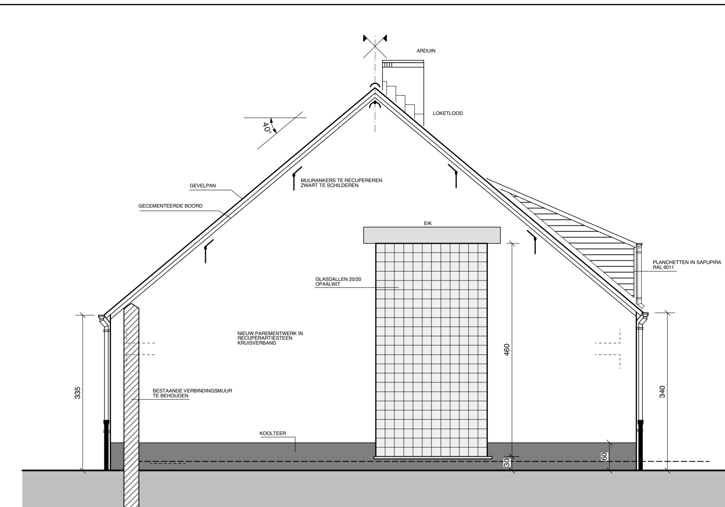
ZIJGEVEL LINKS ontwerp
